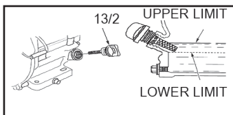
Motoröl-Einfüllschraube
